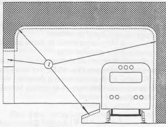
1 — звукопоглощающая облицовка
