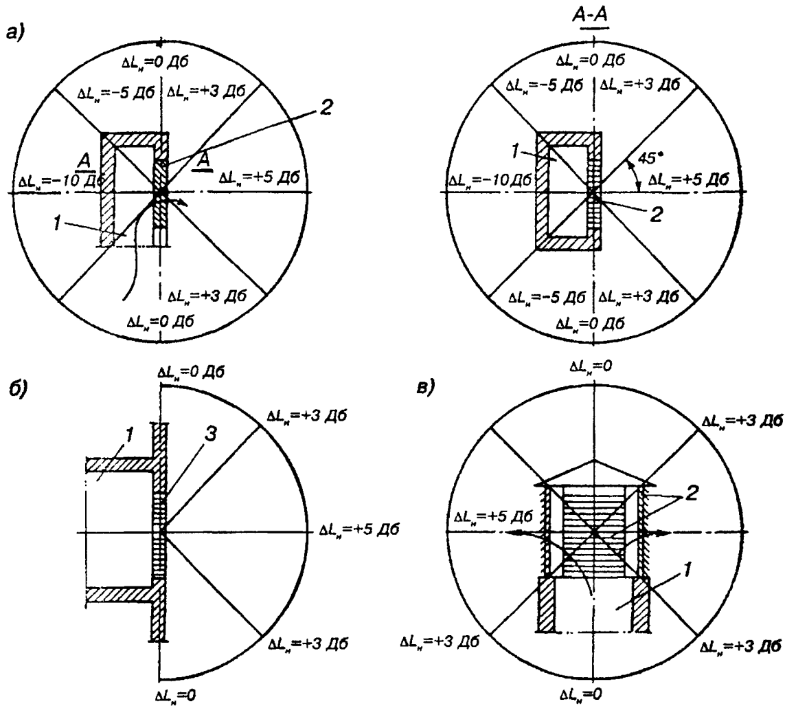
а — всасывание или выпуск в одну сторону через жалюзи; б — то же, через решетку; в — равномерный выпуск во все стороны через жалюзи; 1 — шахта или канал; 2 — жалюзи; 3 — решетка
