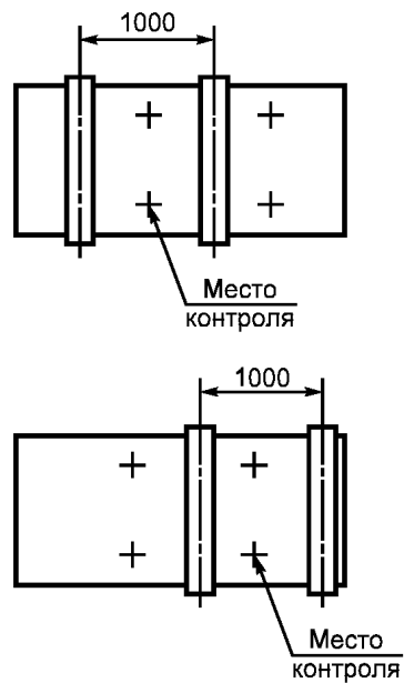
Рисунок А.7 — Схемы испытаний перекрытий и оснований на выпучивание стоечных опор
