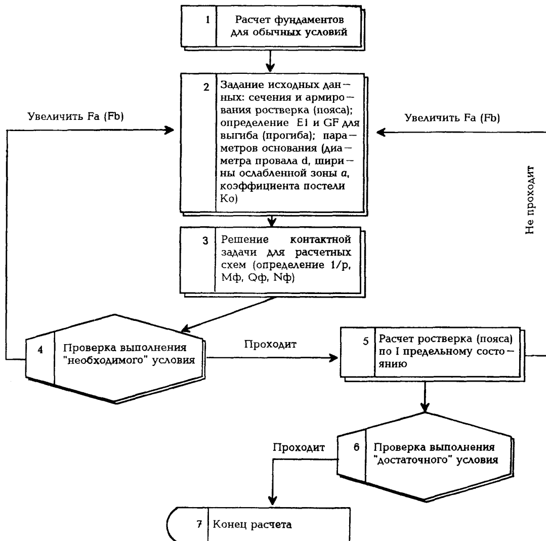
Алгоритм расчета противокарстового железобетонного пояса (ростверка) бескаркасных зданий на воздействие карстового провала
