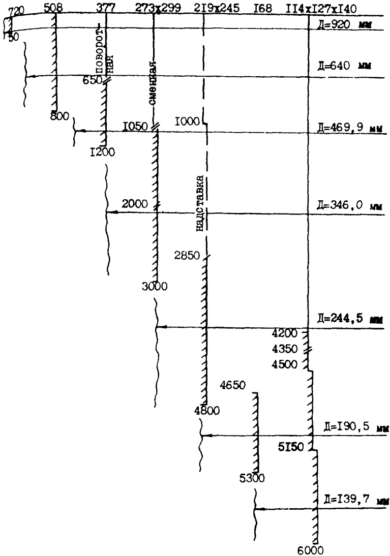
Рис. I. Конструкция скважины (к примеру заполнения табл. 5.2 и 5.3).
