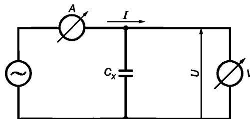
Рисунок 4 — Принципиальная схема измерительной цепи
