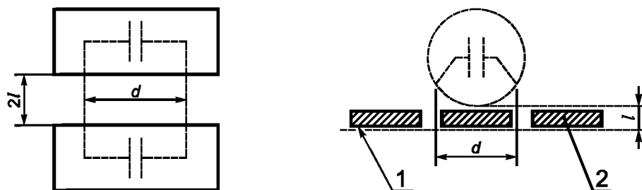
1 — нетравленная медь; 2 — печатная плата.
