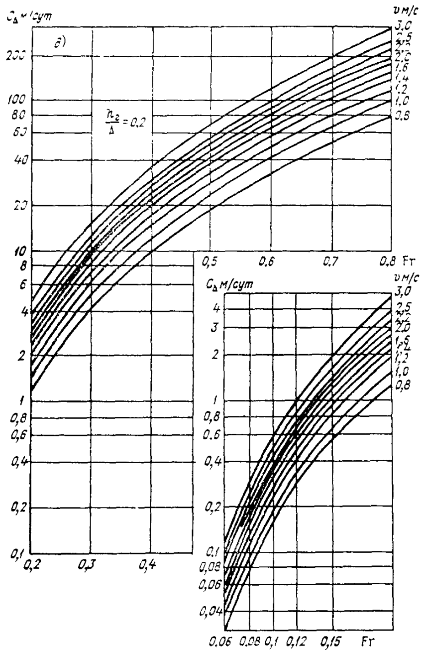
Рис 4.4. Номограммы для расчета скорости движения мезоформ речного русла в зависимости от значения h_2/\Delta .
