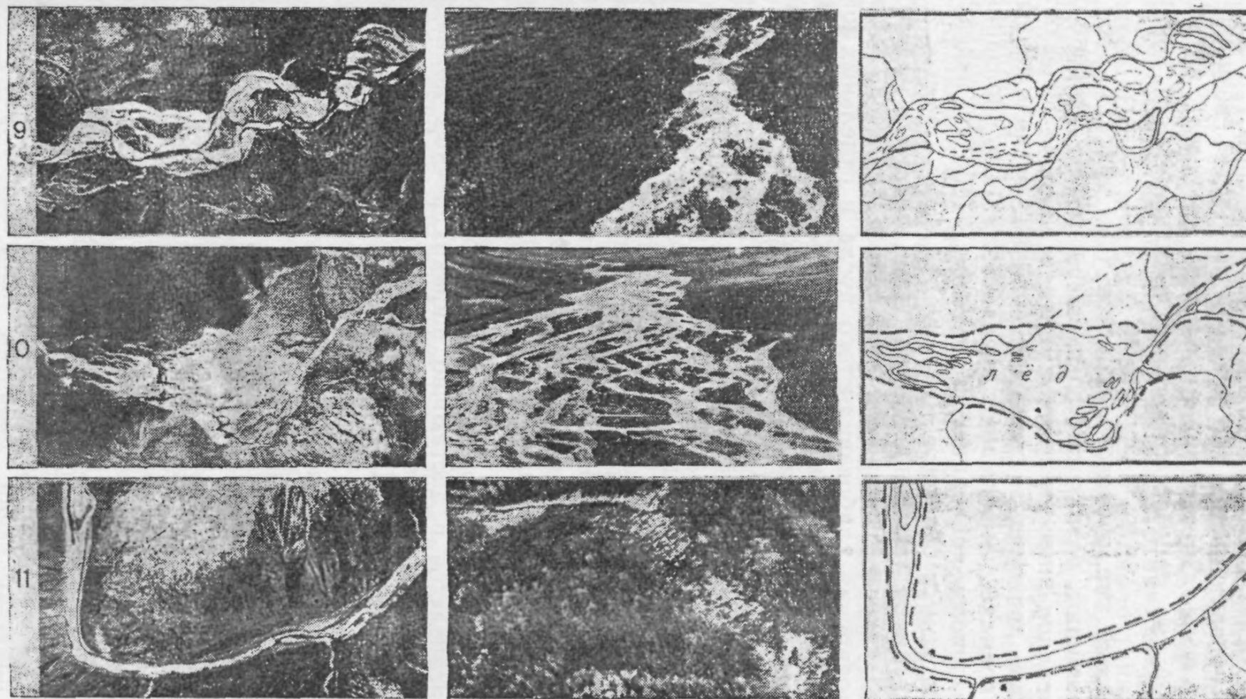
Рис. 3.2. Плановое (а), перспективное (б) и схематическое (в) изображение участков рек зоны БАМ с разными типами руслового процесса.
