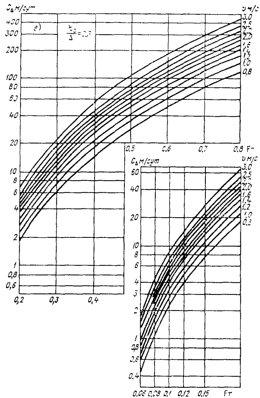
Рис 4.4. Номограммы для расчета скорости движения мезоформ речного русла в зависимости от значения h_2/\Delta .
