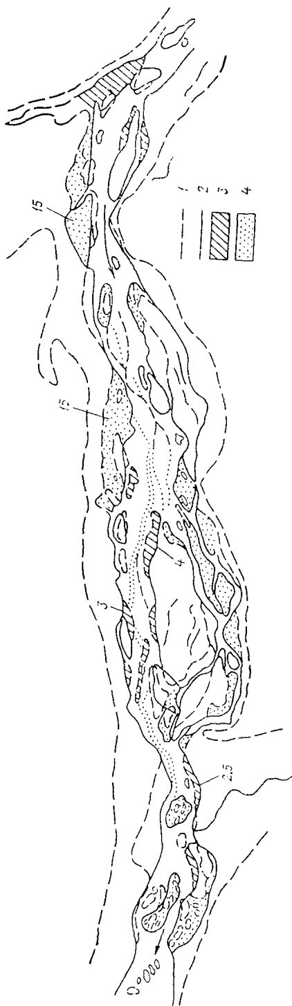
Рис. 4.1. Темпы плановых деформаций на участке русла р. Верхний Сакукан с наледной многорукавностью, м. год. 1 — съемка 1961 г.; 2 — съемка 1975 г.; 3 — размыв; 4 — намыл.
