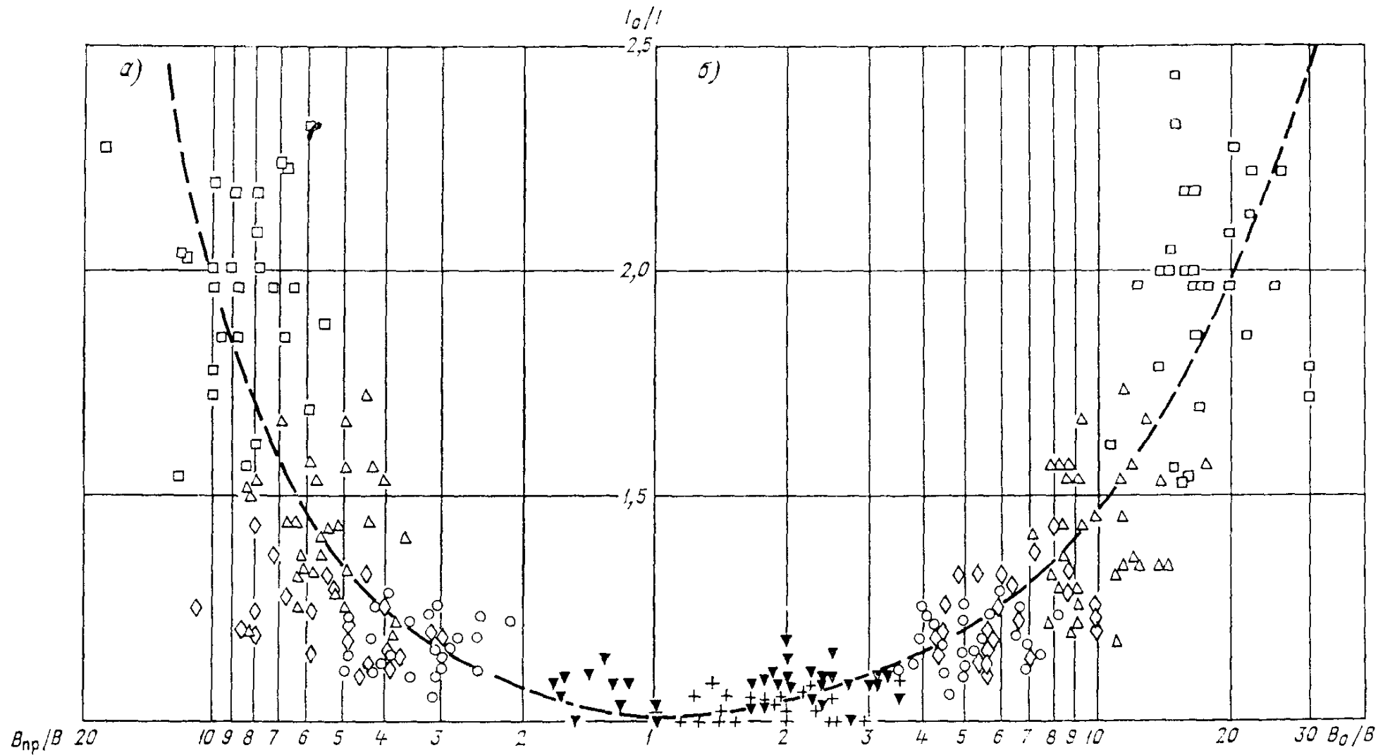
Рис. 3.6. Связь типов руслового процесса. a — с относительными уклонами I_0/l и ширинами пояса руслоформирования B_{np}/B ; b — с относительными уклонами I_0/l и ширинами дна долины B_0/B .
