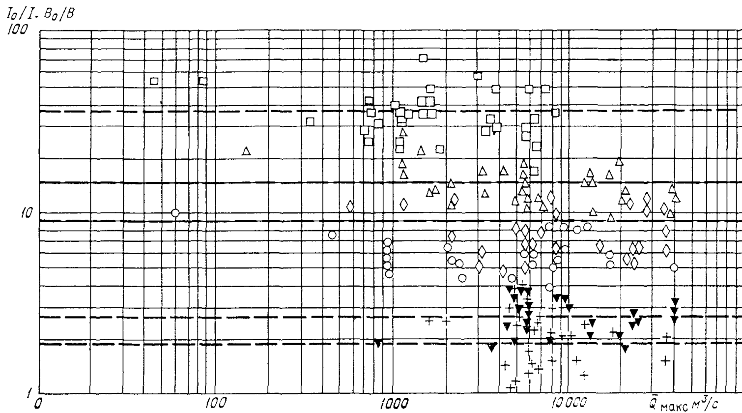
Рис. 3.7. Критеральный график типов руслового процесса.
