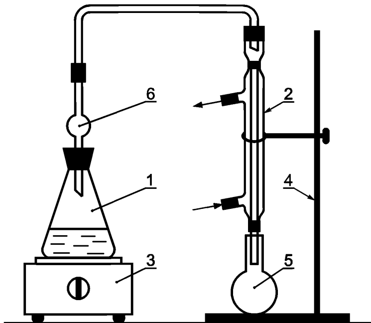
1 — колба с исследуемым жиром; 2 — прямооточный холодильник; 3 — электроплитка с регулятором нагрева; 4 — штатив; 5 — колба для дистиллята; 6 — каплеуловитель
