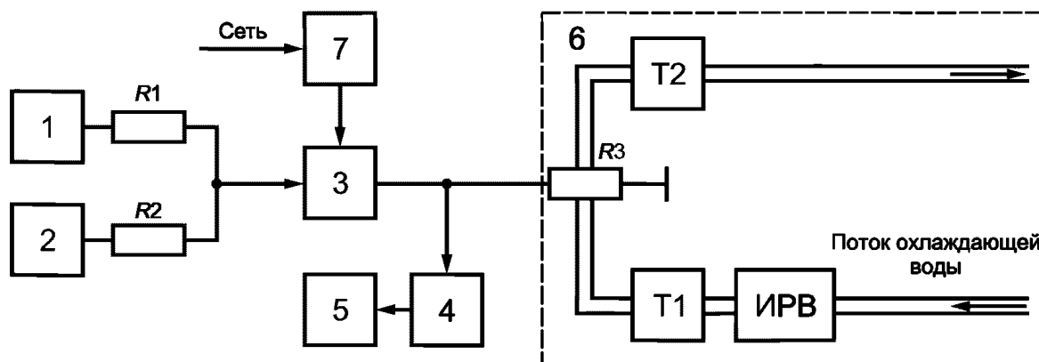
1, 2 — генераторы сигналов НЧ; 3 — передатчик; 4 — элемент связи; 5 — анализатор спектра ВЧ; 6 — эквивалент антенны; R3 — водоохлаждаемый согласованный резистор; T1 , T2 — термометры воды на входе и выходе системы охлаждения; ИПВ — измеритель расхода воды; 7 — ваттварметр (измерительный комплект для измерения потребляемой мощности); R1 , R2 — резисторы сопротивлением (6,8 \pm 0,34) кОм
