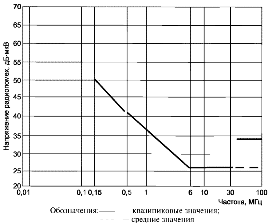
Рисунок 2 — Нормы напряжения радиопомех
