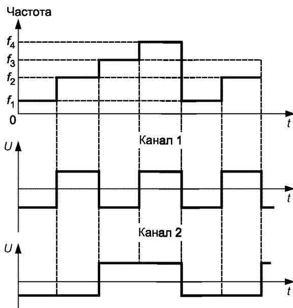
Рисунок 23 — Формирование испытательного сигнала при работе передатчика классом излучения F7В
