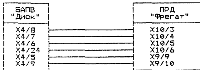
Рис. 5 Схема электрических соединений БАПВ "Диск" с РПД "Фрегат"
