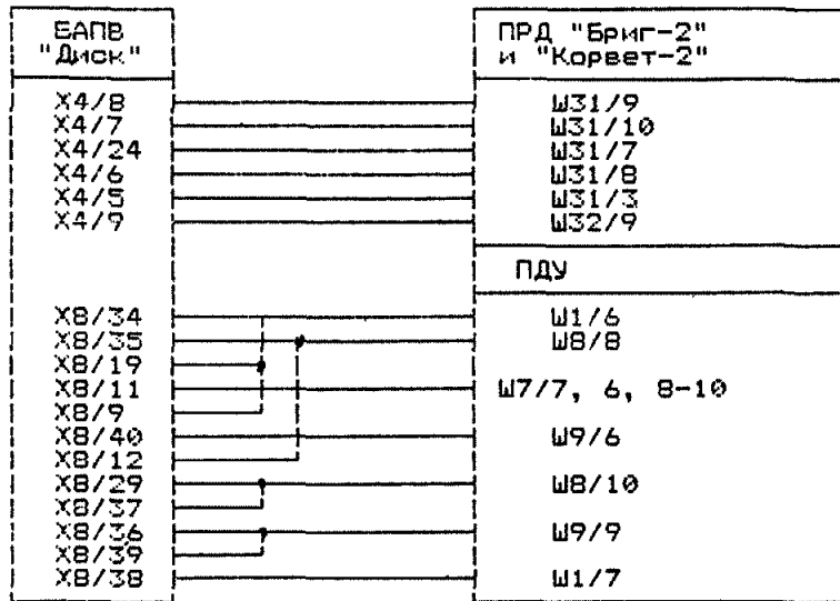
Рис. 4 Схема электрических соединений БАПВ "Диск" с РПД "Бриг-2" и "Корвет-2".
