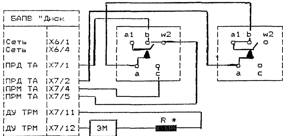
Рис.14 Схема электрических соединений БАПВ "Диск" с телеграфным аппаратом Т-63 и трансмиттером Т53.
