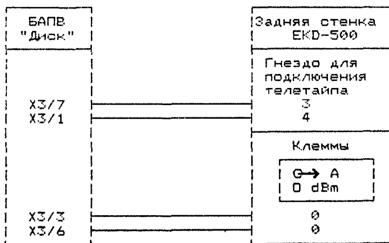
Рис. 10 Схема электрических соединений БАПВ "Диск" с РПУ "ЕКD-500"
