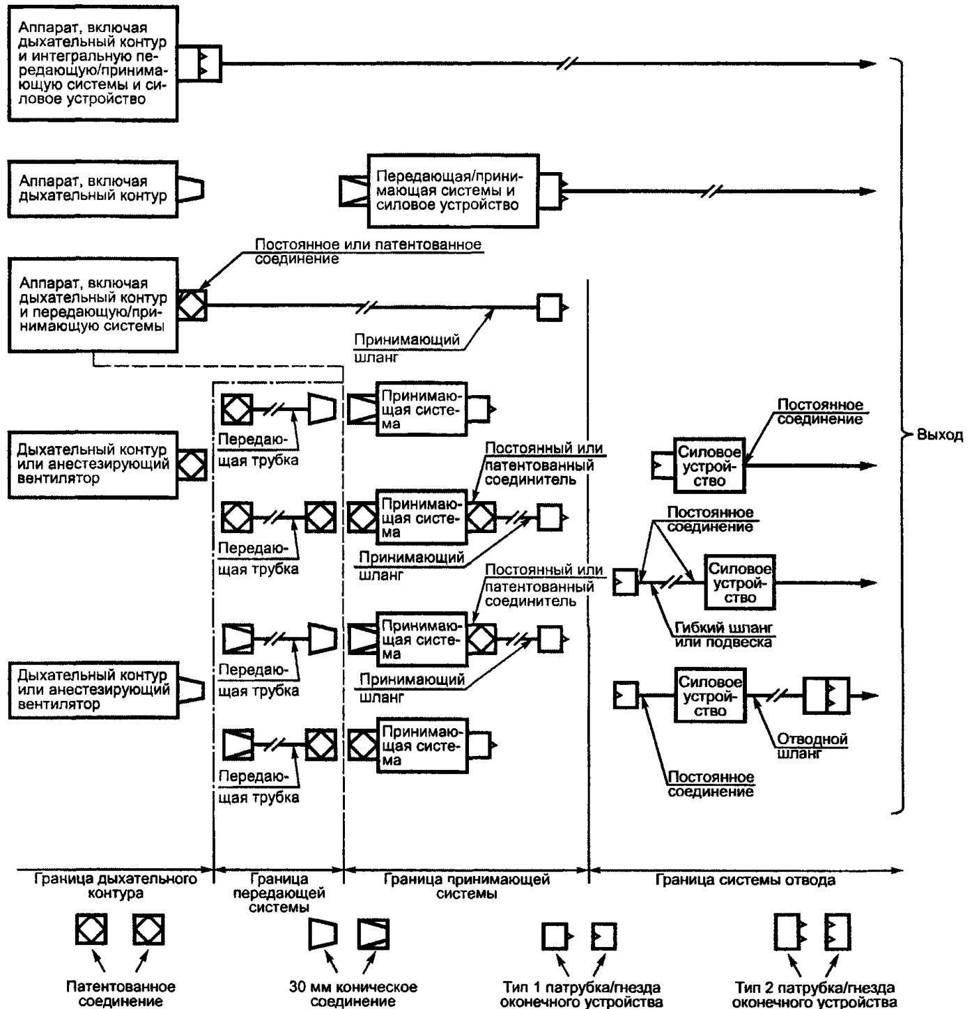
Рисунок 1 — Схема типичных соединений СВГС
