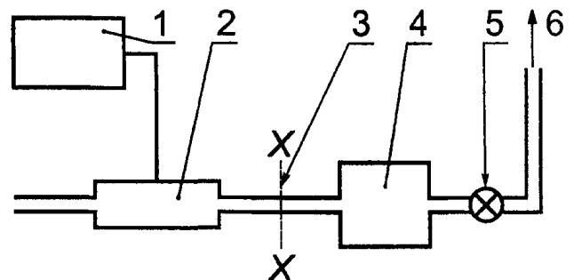
Рисунок В.1 — Схема испытаний на индуцированный поток
