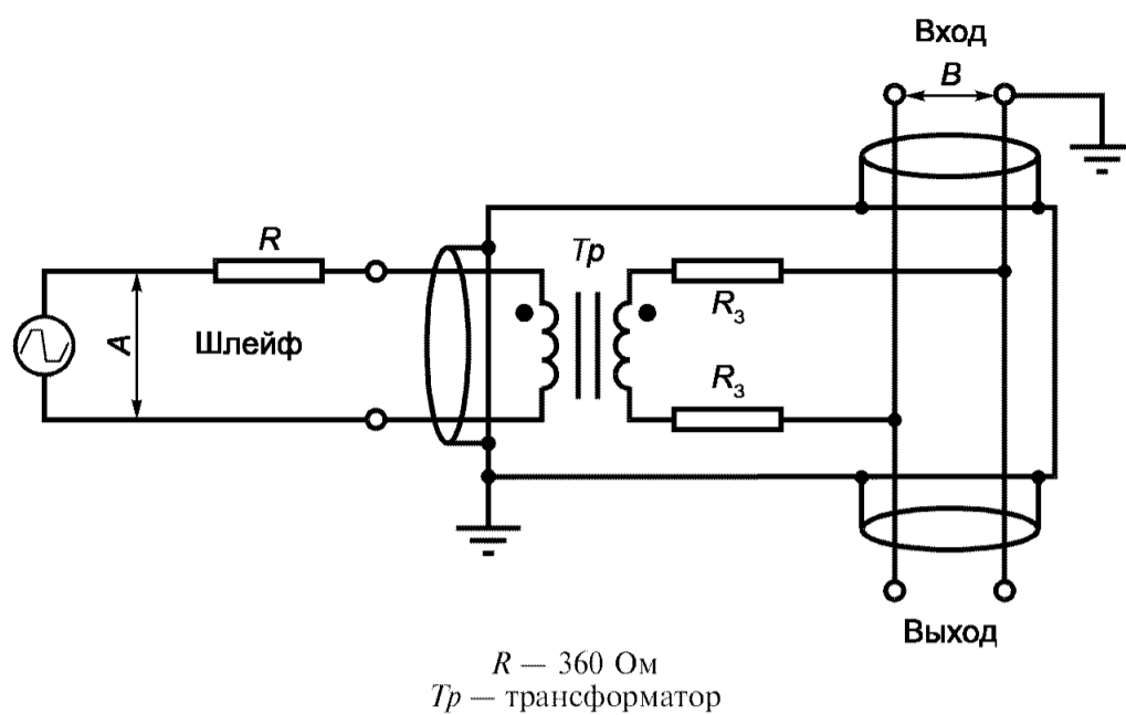
Рисунок 3 — Схема измерения выходного сигнала
