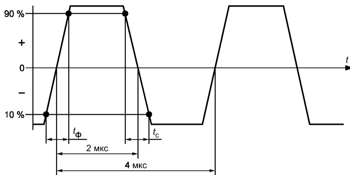
Рисунок 4 — Форма и параметры входного сигнала
