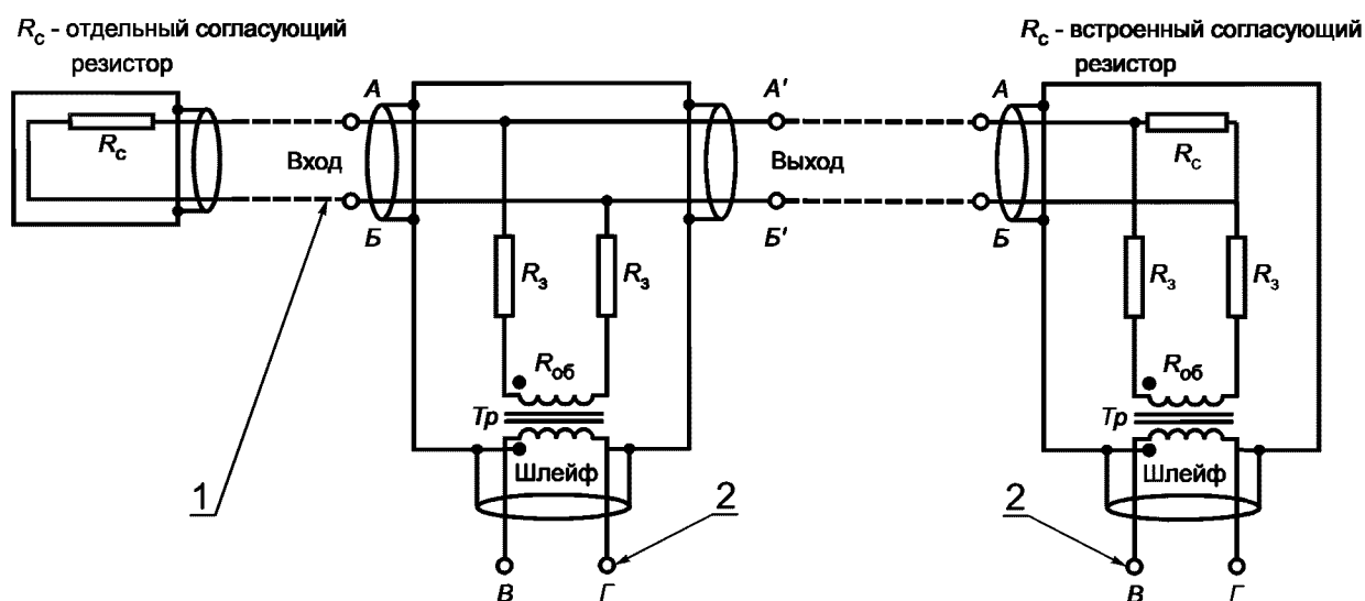
1 — магистральная шина; 2 — кабель шлейфа
