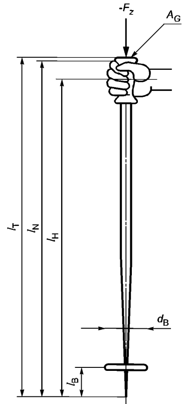
Рисунок 2 — Условное обозначение размеров горнолыжной палки
