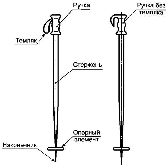
Рисунок 1 — Элементы горнолыжной палки и термины
