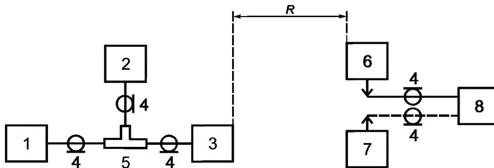
1 — генератор сигналов высокочастотный; 2 — частотомер электронно-счетный; 3 — вспомогательная передающая антенна; 4 — соединительные кабели; 5 — тройник; 6 — испытываемая антенна; 7 — измерительная антенна; 8 — измеритель уровней сигналов телевидения и радиовещания; R — расстояние между вспомогательной и испытываемой антеннами
