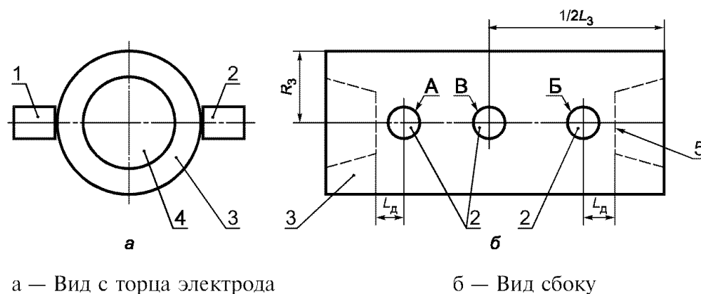
Рисунок В.1 — Расположение мест контроля в заготовках
