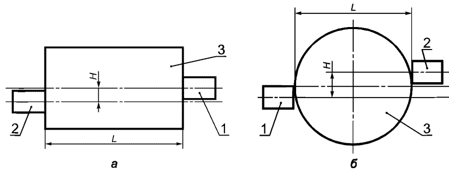
а — Изделия с плоскопараллельными поверхностями
