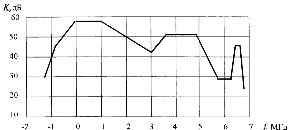
Рисунок 5.1 — Кривая защитных отношений для системы вещательного телевидения
