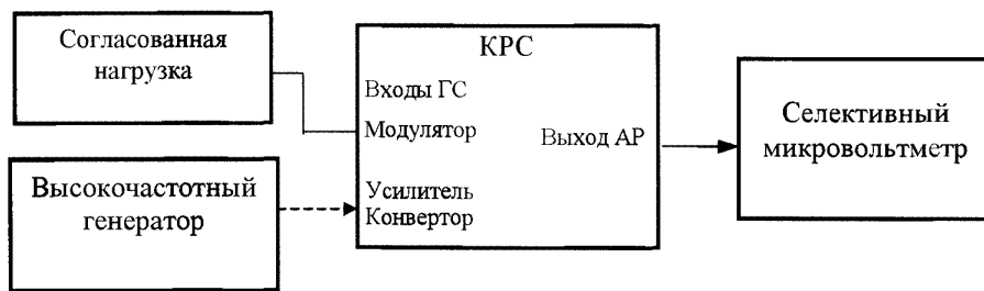
Рисунок 7.4 — Структурная схема для определения отношения радиосигнала изображения к шуму
