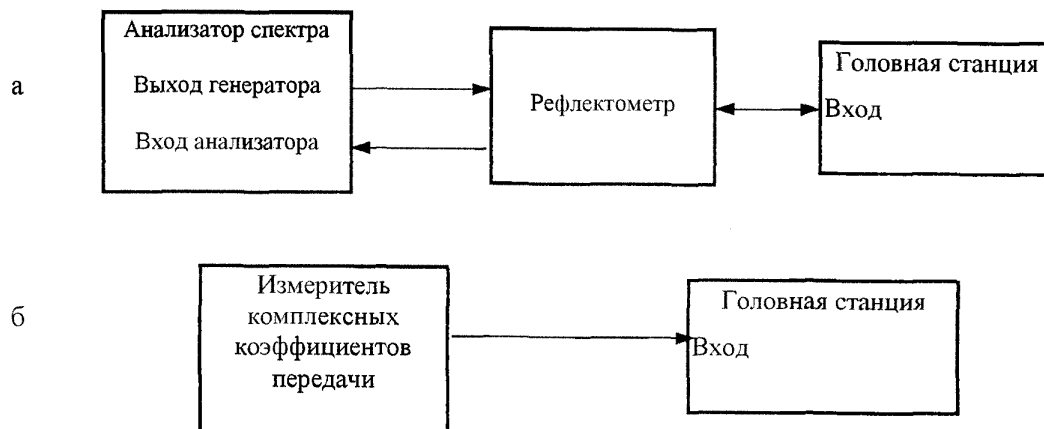
Рисунок 7.15 — Структурная схема для измерения затухания несогласованности
