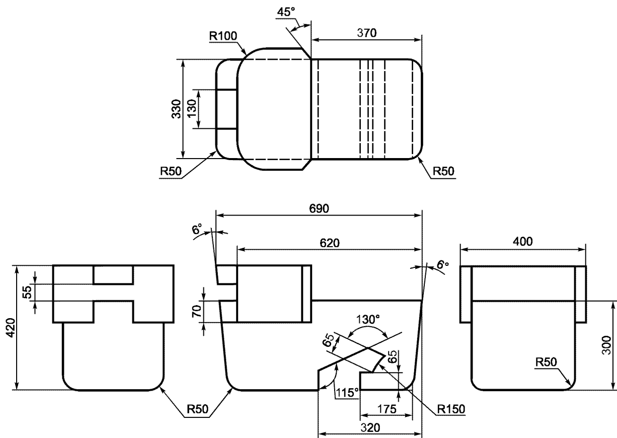
Рисунок 17.1 — Спецификация зажимного приспособления
