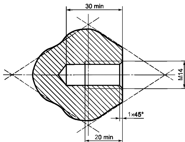
Рисунок 6.4 — Стопорное устройство (овальный наконечник)
