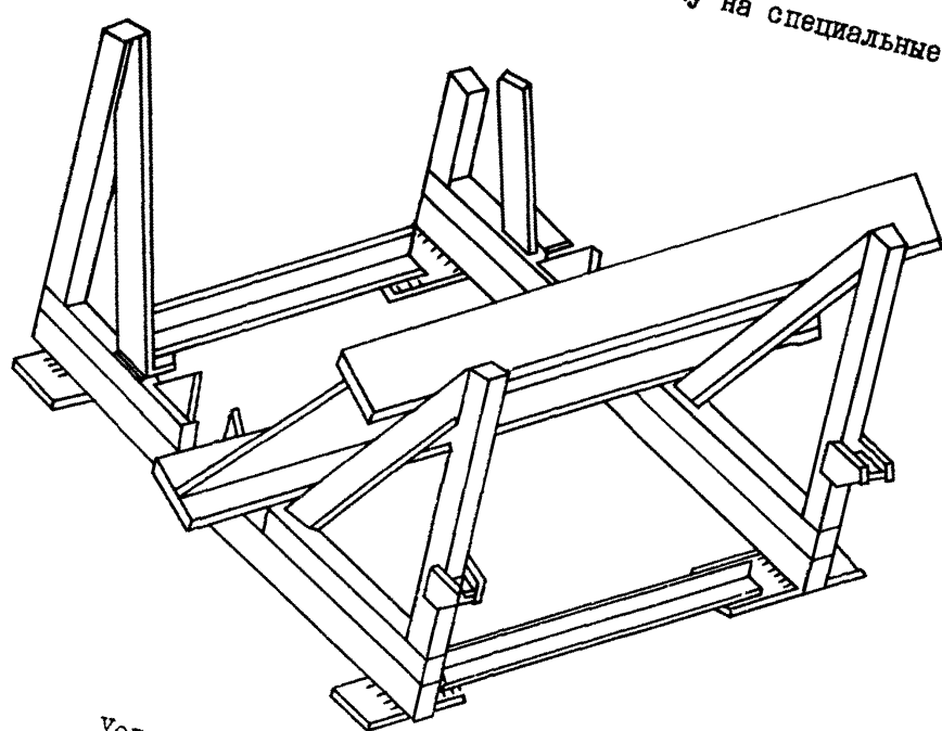
Установка балок для сварки в лодочку
