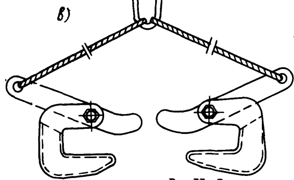
Рис. 11. Захват: а - крючковой для перевозки цистерн; б - для труб; в - для листового металла
