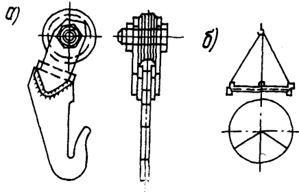
Рис. 19. Тросовый захват для транспог- тировки днищ и резервуаров: а - крюк захвата; б - схема строповки днища захватом
