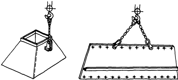
Рис.26. Строповка элементов бункеров серьями
