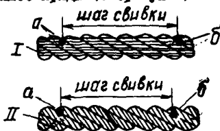
Схема свивки каната: I - крестовой; II - односторонней
