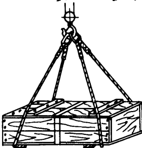
Рис.22. Строповка ящиков стропами
