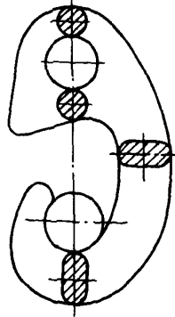
Рис.4. Крюк
