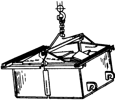
Рис.20. Строповка тары цепями
