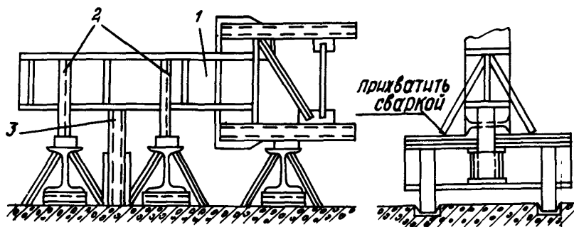
Крепление колонны на стеллажах распорками: 1 - колонна; 2 - распорка; 3 - инвентарная стойка
