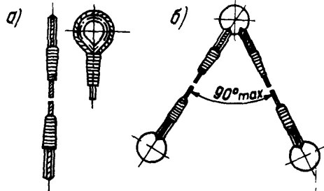
Рис.6. Строп канатный:
