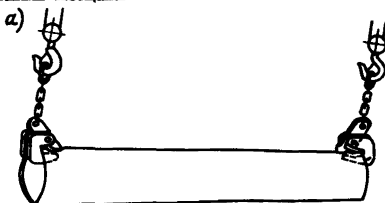
Рис.1. Транспортировка и кантовка листовых деталей самовхватными клещами
