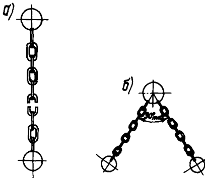
Рис.8. Строп цепной:
