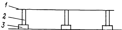
Рис.2. Стоечные ограждения:
