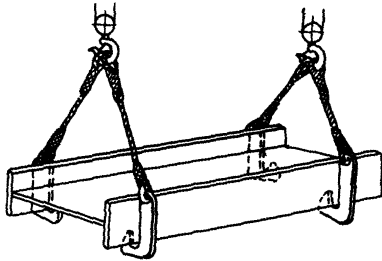
Рис.12. Транспортировка балок стропами с крюками
