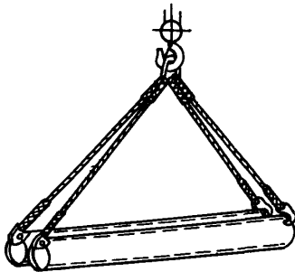
Рис.24. Строповка труб стропами с кольцами
