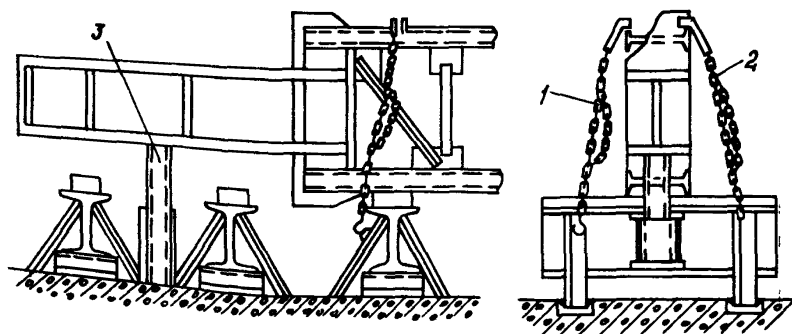
Крепление колонны расчалками: 1 - расчалка; 2 - карабин; 3 - инвентарная стойка
