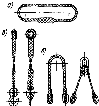
Рис. 17. Специальные строповочные тросы и стропы: а - универсальный; б - облегченный, с петлями и крючками; в - облегчен- ные с кольцами
