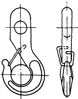
Рис.5. Крюк
