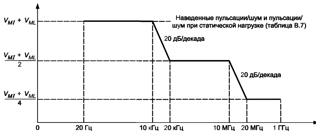
Рисунок В.46 — Уровни восприимчивости модуля к помехам
