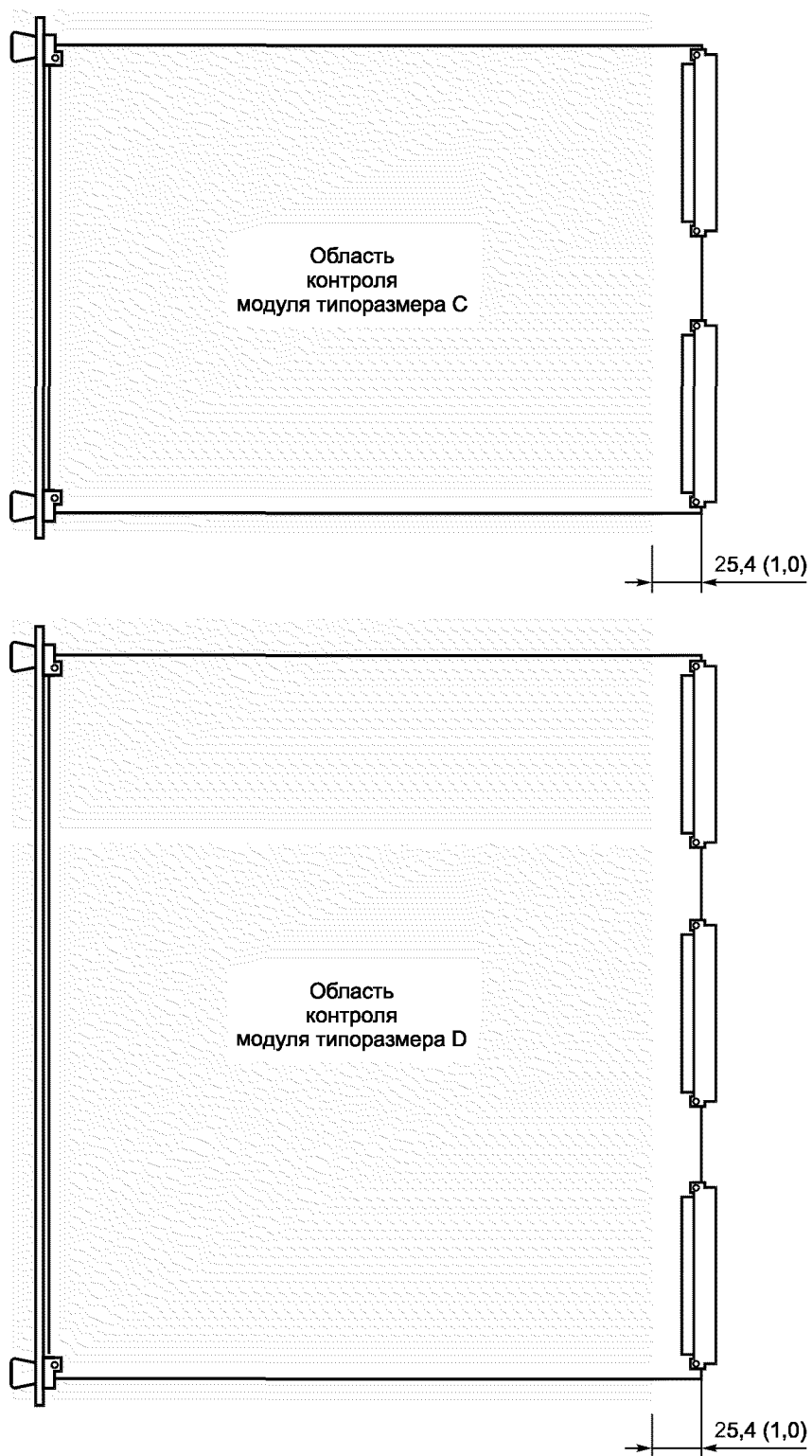
Рисунок В.52 — Области контроля ЭМС для модулей типоразмеров C и D
