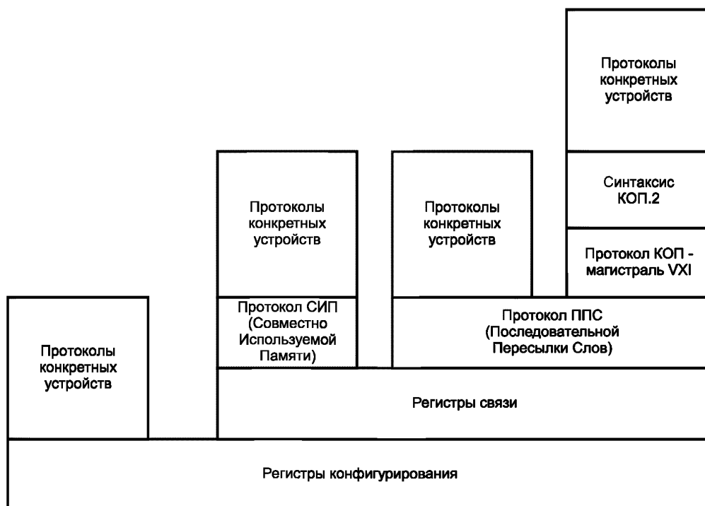
Рисунок С.2 — Уровни протоколов информационного обмена VXI
