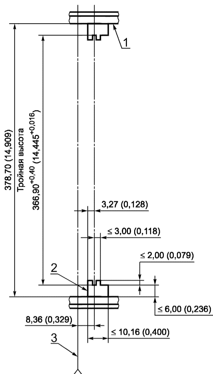
1 — горизонтальный элемент; 2 — направляющая; 3 — межмодульная разделительная плоскость
