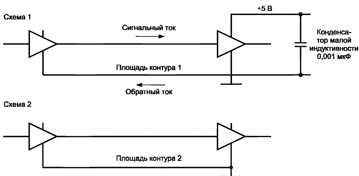
Рисунок II.1 — Типичные логические схемы
