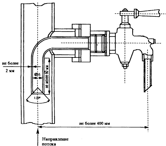
Рис. Устройство для отбора проб из напорных трубопроводов.
