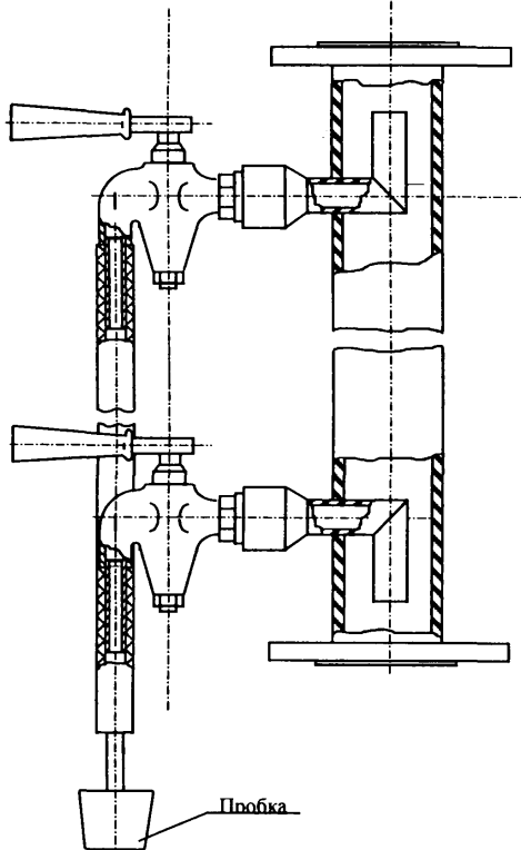
Устройство для отбора проб из приемных трубопроводов
