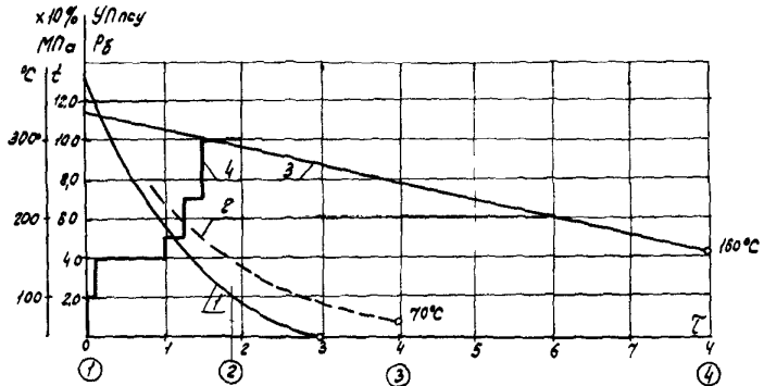
Рис.7. График-задание останова котла с расхолаживанием барабана и главного паропровода:
