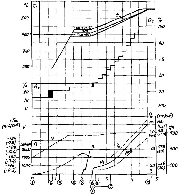
Рис.4. График-задание пуска энергоблока из неустывшего состояния (температура металла верха ЦВД в зоне регулирующей ступени 290-330 ^{\circ}\text{C} , продолжительность простоя 24-31 ч).
