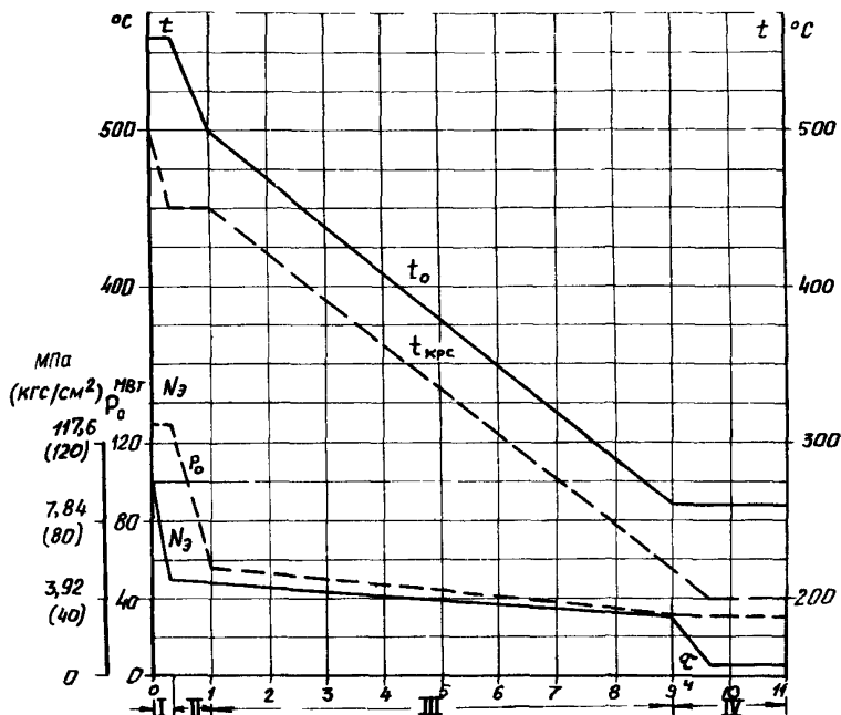
Рис.6. График-задание останова энергоблока с расхолаживанием турбины:
