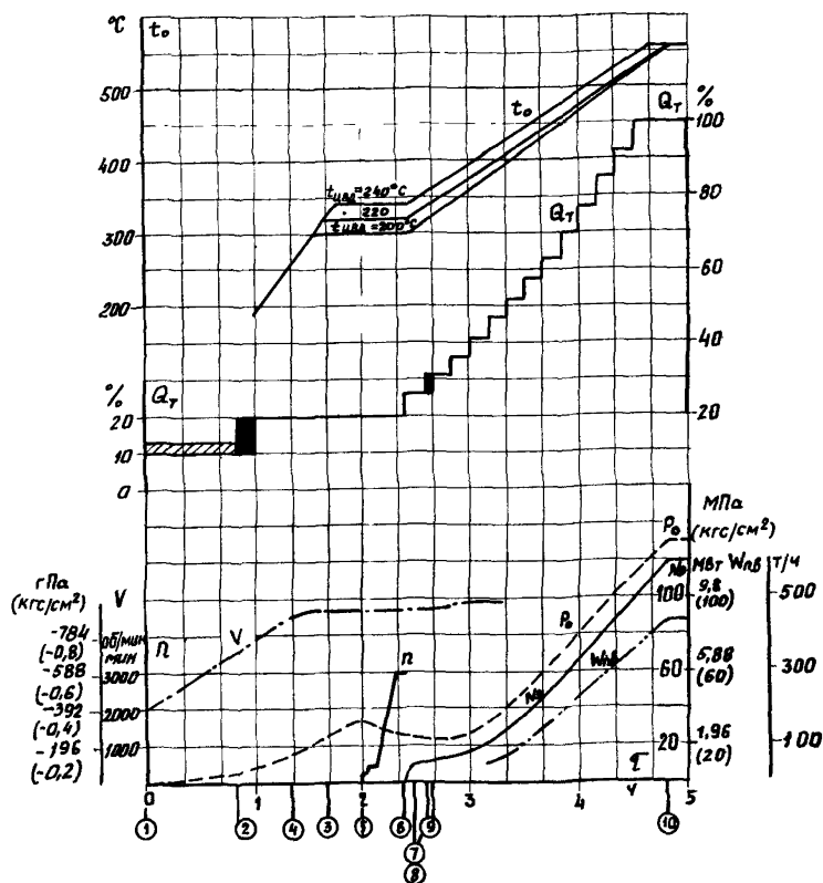
Рис.3. График-задание пуска энергоблока из неустывшего состояния (температура металла верха ЦВД в зоне регулирующей ступени 200-240 ^{\circ}\text{C} , продолжительность простоя 48-55 ч);
