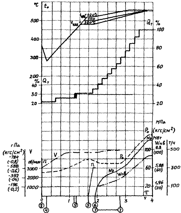
Рис.5. График-задание пуска энергоблока из горячего состояния (температура металла верха ЦВД в зоне регулирующей ступени 380-420^{\circ}\text{C} , продолжительность простоя 8-10ч).
