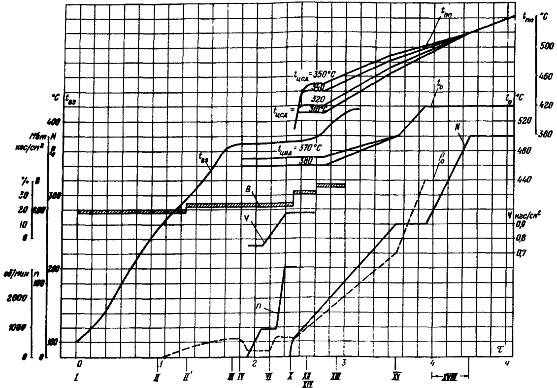
Рис. 6. График-задание пуска блока из неостывшего состояния (температура паровпуска ЦВД 370-380°C, температура паровпуска ЦСД 310-350°C, продолжительность простоя 24-30 ч)
