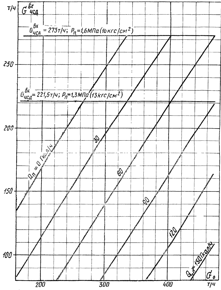
Рис. 18 ТИПОВАЯ ЭНЕРГЕТИЧЕСКАЯ ХАРАКТЕРИСТИКА ТУРБОАГРЕГАТА РАСХОД ПАРА НА ВХОДЕ В ЧСД ПРИ РЕЖИМАХ С РЕГУЛИРУЕМЫМИ ОТБОРАМИ
