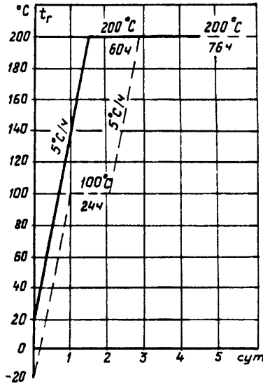
Рис. 1. Контрольный график сушки футеровки и железобетонной дымовой трубы и газоходов:
