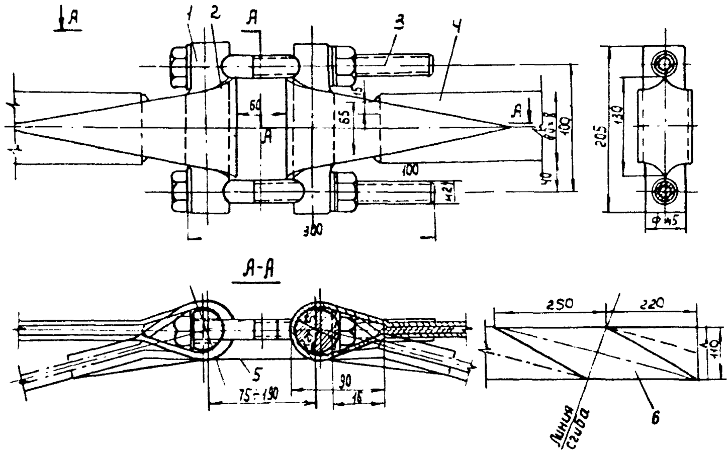
Рис. 5. Конструкция двухшарнирного стыкового замка:
