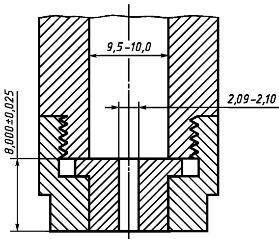
Рисунок 9 — Фильтра
