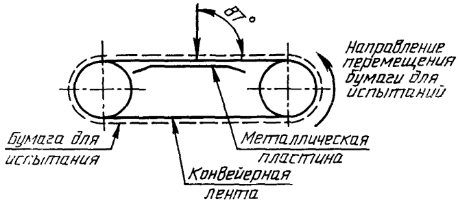
Рисунок 1 — Схема испытательного устройства
