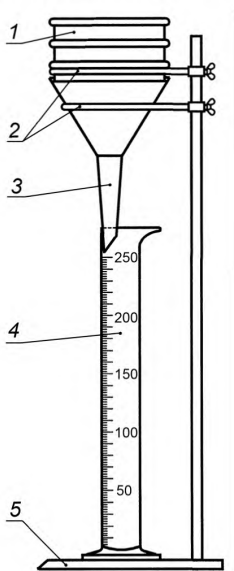
1 — сито; 2 — кольцо; 3 — стеклянная воронка; 4 — мерный цилиндр; 5 — штатив
