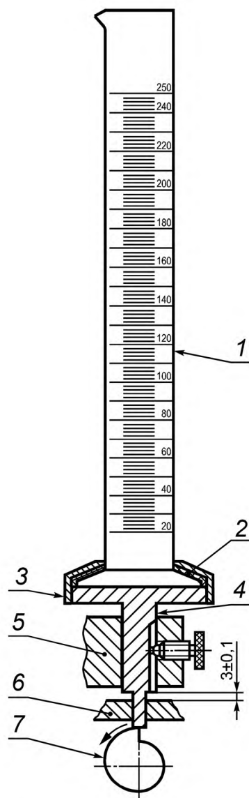
1 — мерный цилиндр; 2 — резиновая втулка; 3 — держатель для мерного цилиндра; 4 — ось; 5 — втулка; 6 — наковальня; 7 — кулачок
