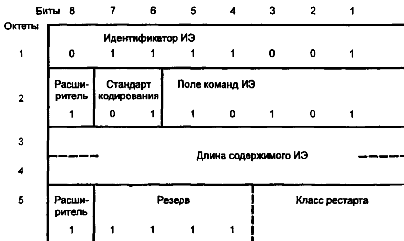
Рисунок 16 — Формат ИЭ «Индикатор рестарта»
