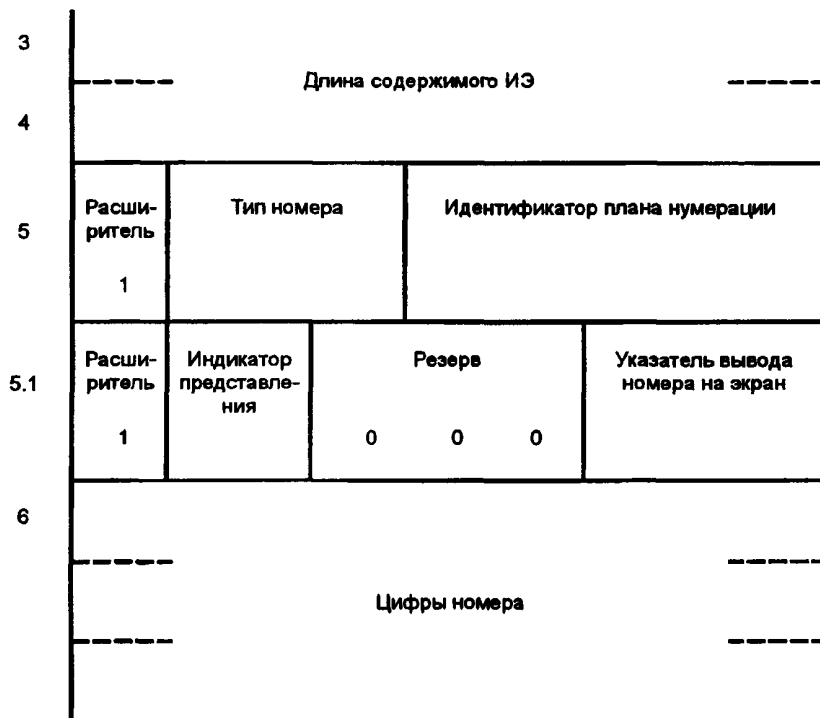
Рисунок 9 — Формат ИЭ «Номер вызывающей стороны»
