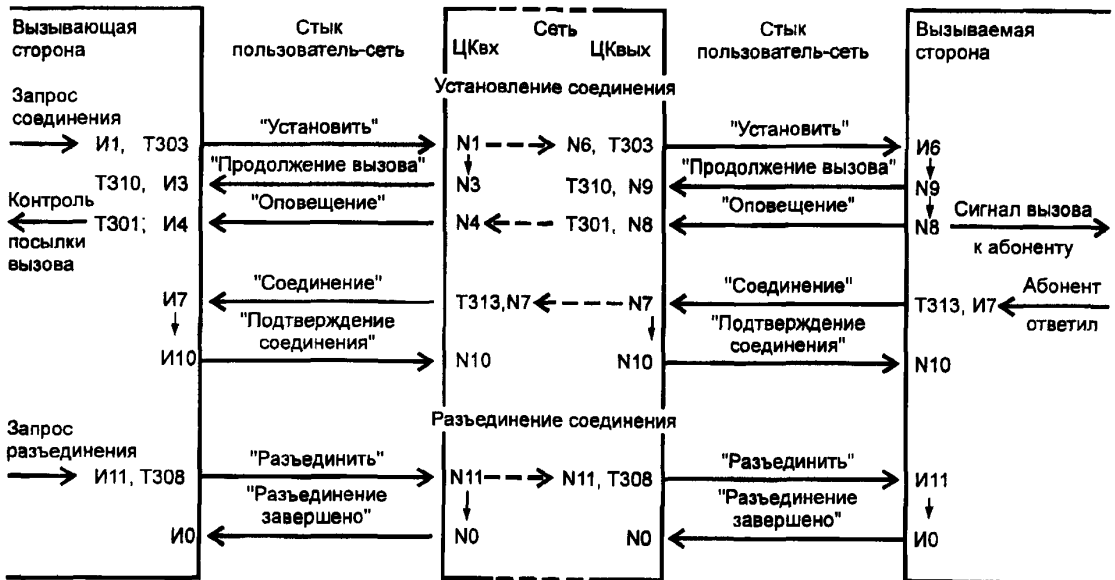
Рисунок 18 — Последовательность передачи сообщений
