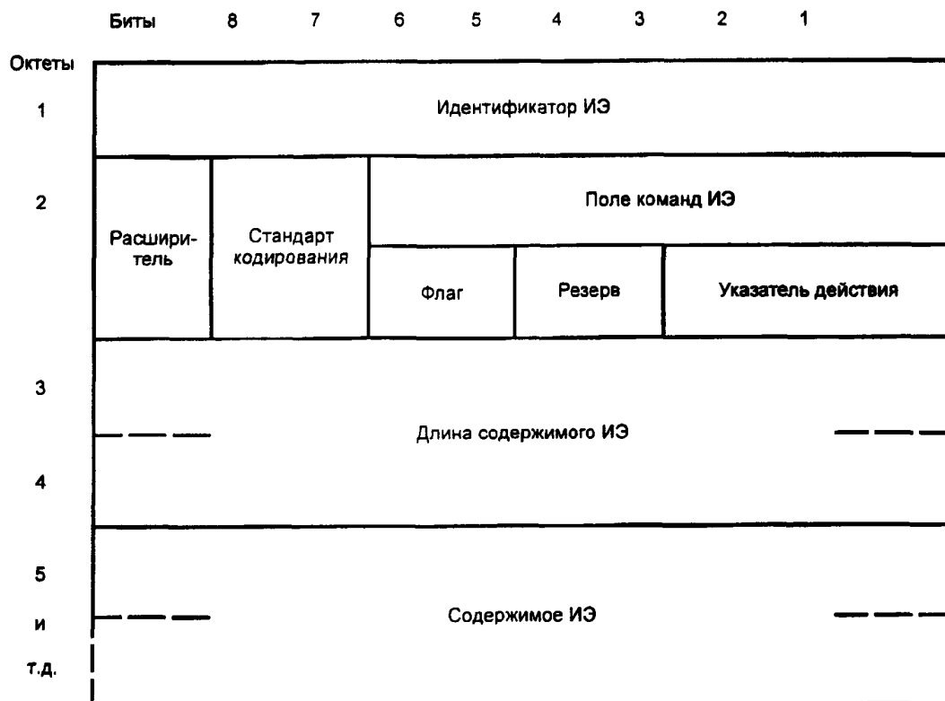
Рисунок 3 — Структура формата ИЭ
