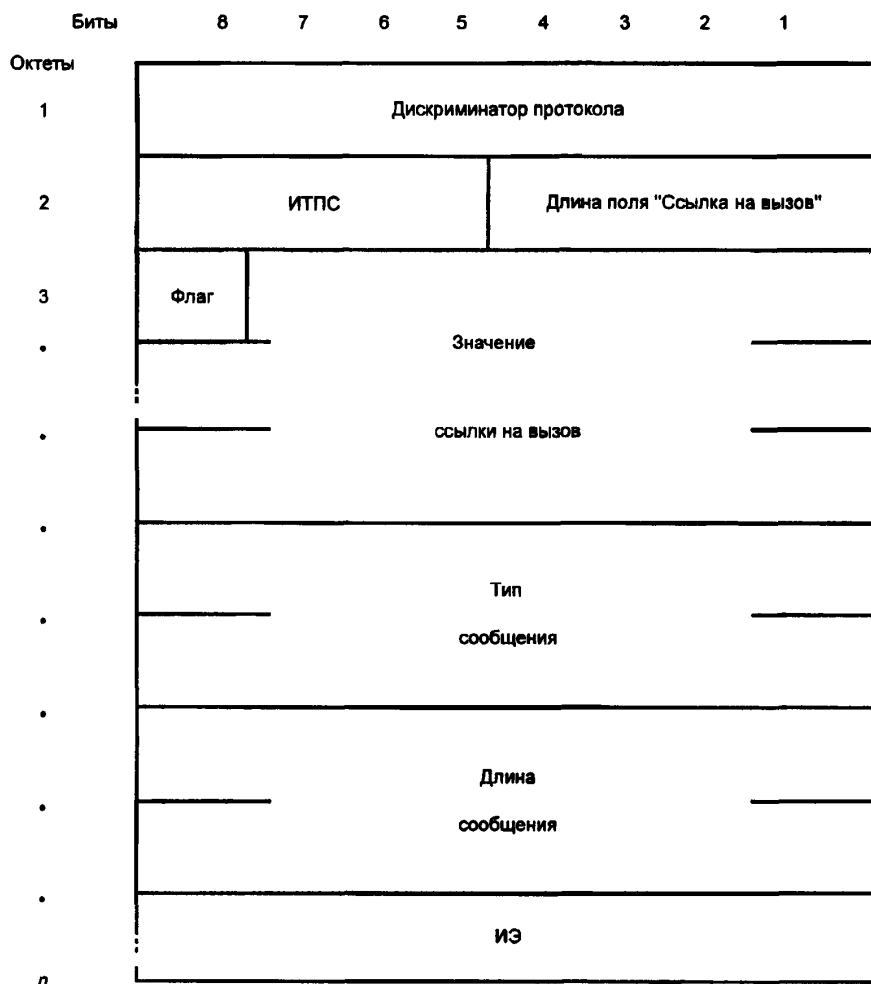
Рисунок 1 — Структура формата
