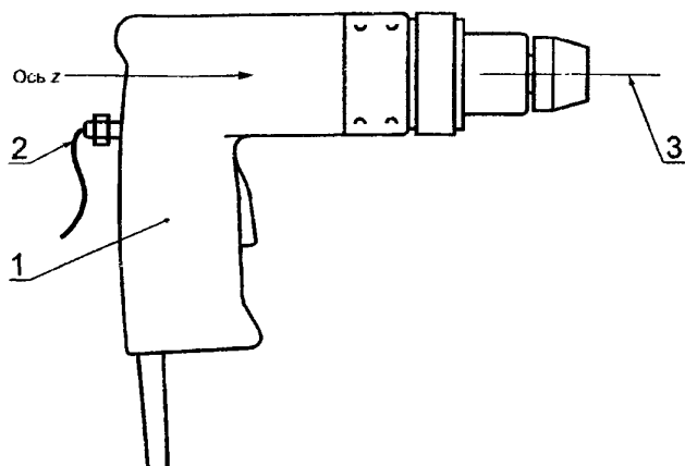
Рисунок 1 — Направление измерений, пример расположения и крепления вибропреобразователя
