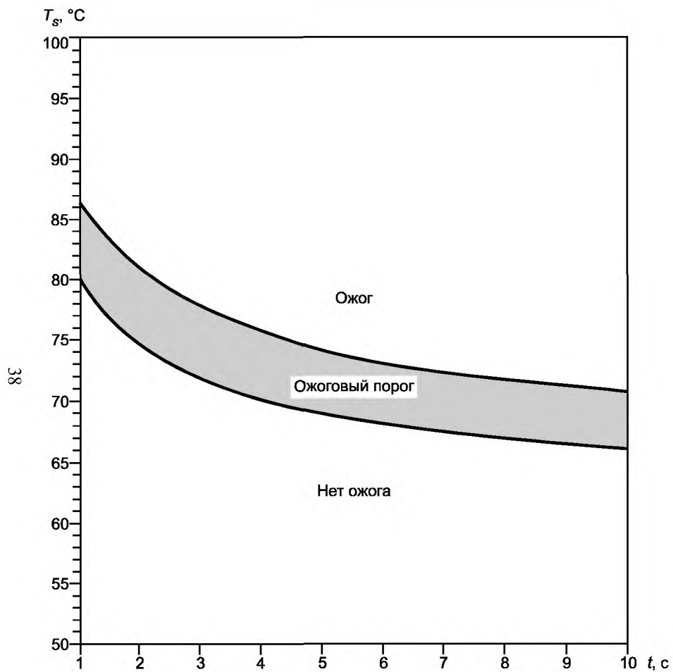
Рисунок 4 — Область ожогового порога при соприкосновении кожи с гладкой горячей поверхностью из керамики, стекла и камня
