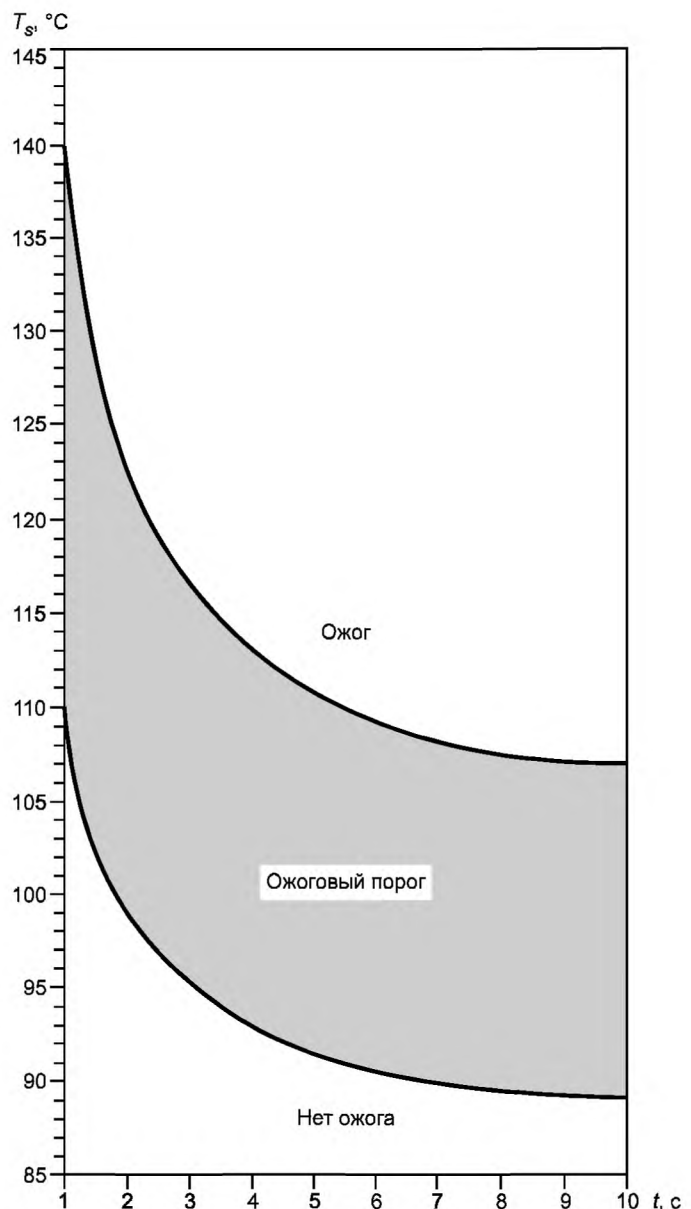
Рисунок 6 — Область ожогового порога при соприкосновении кожи с гладкой горячей поверхностью из дерева
