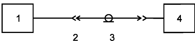
1 — измеритель КСВН; 2 — коаксиальный переход; 3 — фидер антенны; 4 — антенна
