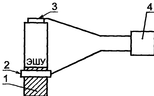
1 — рукоятка; 2 — медная фольга; 3 — электроды; 4 — высоковольтный источник напряжения
