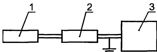
1 — источник питания; 2 — стационарное ЭШУ; 3 — вольтметр
