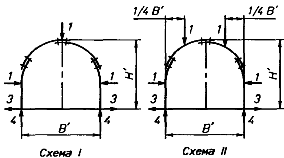
б) Четырехзвенные арочные крепи
