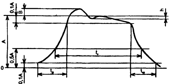
Рисунок 12 — Форма сигнала оптического излучения в ВОСРП
