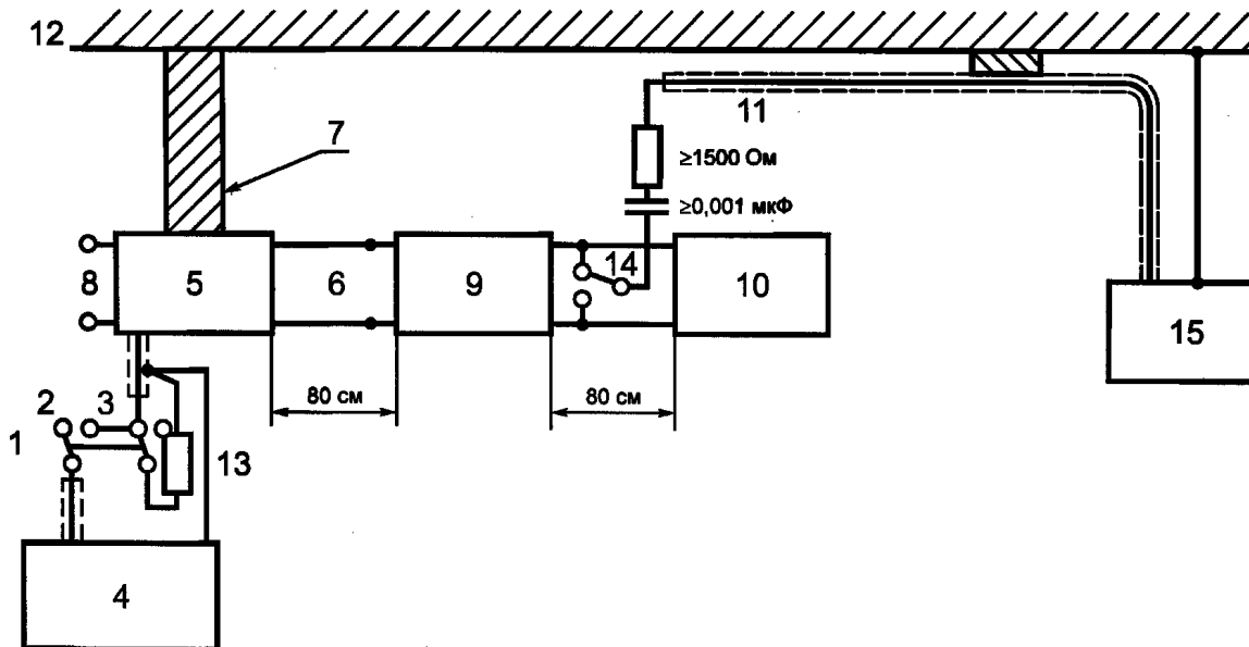
1 — переключатель измерителя радиопомех; 2 — положение переключателя, соответствующее измерениям на нагрузке; 3 — положение переключателя, соответствующее измерениям в сети электропитания; 4 — измеритель радиопомех; 5 — эквивалент сети; 6 — подключение эквивалента сети ко входу СБП; 7 — заземляющая шина (отношение длины к ширине 3:1); 8 — подключение к сети электропитания; 9 — СБП; 10 — нагрузка; 11 — пробник напряжения; 12 — пластина заземления; 13 — нагрузочный резистор (50 Ом); 14 — переключатель пробника напряжений; 15 — альтернативное место размещения измерителя радиопомех
