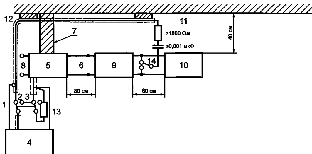
1 — переключатель измерителя радиопомех; 2 — положение переключателя, соответствующее измерениям на нагрузке; 3 — положение переключателя, соответствующее измерениям в сети электропитания; 4 — измеритель радиопомех; 5 — эквивалент сети; 6 — подключение эквивалента сети ко входу СБП; 7 — заземляющая шина (отношение длины к ширине 3:1); 8 — подключение к сети электропитания; 9 — СБП; 10 — нагрузка; 11 — пробник напряжения; 12 — пластина заземления; 13 — нагрузочный резистор (50 Ом); 14 — переключатель пробника напряжений
