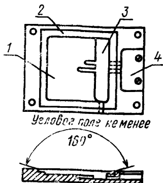
Рисунок 2 — Конструкция из одного элемента
