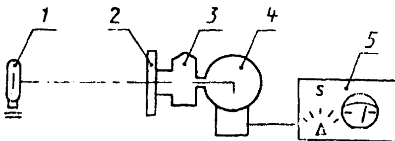
1 — нормированный источник света; 2 — молочное стекло; 3 — испытуемый фотоаппарат; 4 — светочувствительный блок; 5 — контрольно-измерительный прибор
