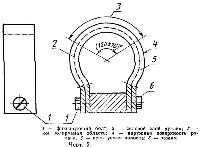
Схема установки образца (метод 2)
