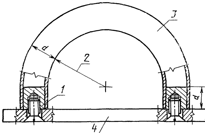
Схема установки рукава (метод 1)
