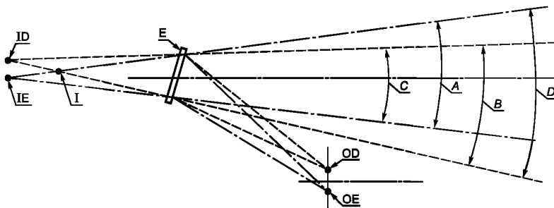
E — внутреннее зеркало заднего вида; OD , OE — глаза водителя; ID , IE — виртуальное монокулярное изображение; I — виртуальное ambiнокулярное изображение; A — угол обзорности левого глаза; B — угол обзорности правого глаза; C — бинокулярный угол обзорности; D — ambiнокулярный угол обзорности
