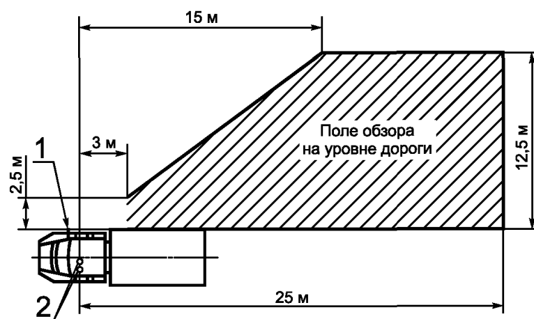
1 — зеркало заднего вида; 2 — окулярные точки водителя
