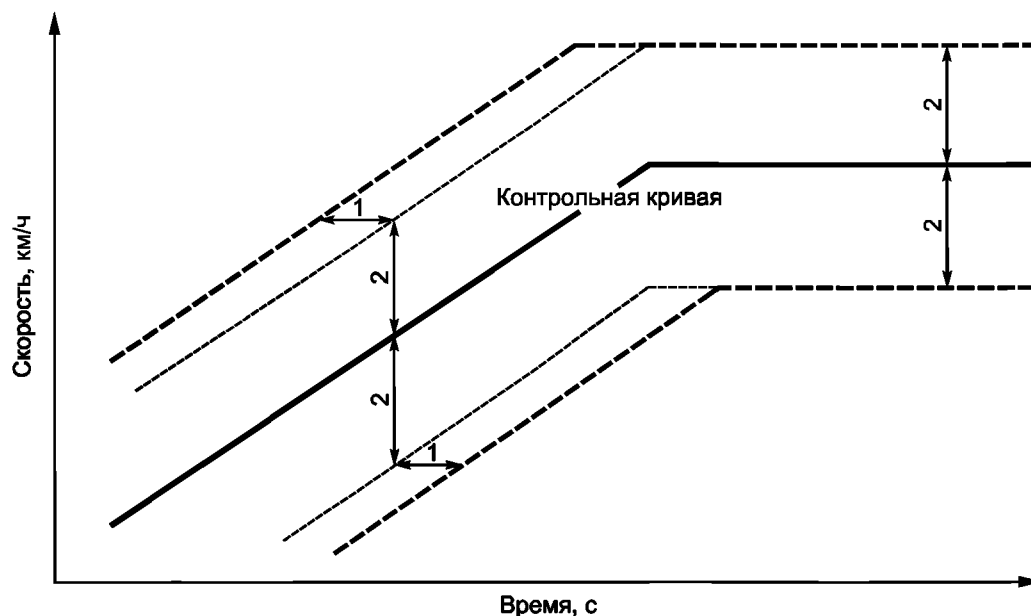
Рисунок 4 — Допустимое отклонение скорости
