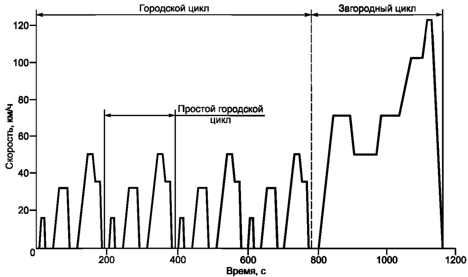
Рисунок 1 — Последовательность испытаний транспортных средств категорий M_1 и N_1
