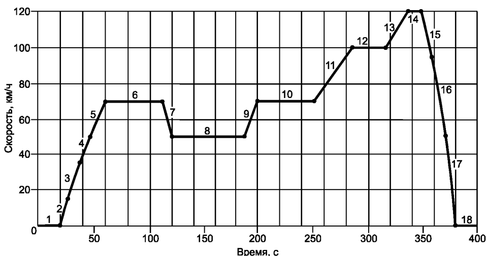
Рисунок 3 — Загородный цикл (400 с)
