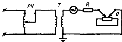
PУ —регулирующее устройство; T —трансформатор; R —сопротивление 0,5 МОм; O —образец из карбо- лита с нанесенной пленкой испытуемой эмали.
