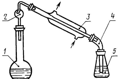
1 — колба Кьельдаля; 2 — каплеуловитель, 3 — холодильник, 4 — аллонж, 5 — приемная колба
