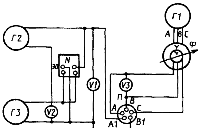
А В С А1 В1 — зажимы синхроскопа Г1 — трехфазный генератор Г2 Г3 — однофазные генераторы V1 V2 V3 — вольтметры среднего квадратического значения класса I Ф — фазорегулятор П — проверяемый синхроскоп ЭО — осциллограф электронный точечной
