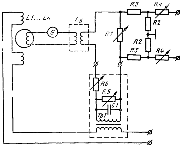
R_4 —регулируемое сопротивление; C_1 —емкость, T_{р1} —трансформатор, L_1 L_n —набор регулировочных индуктивностей
