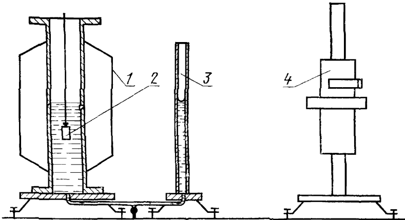
1—преобразователь расхода, 2—груз; 3—калиброванный стеклянный сосуд; 4—катетометр
