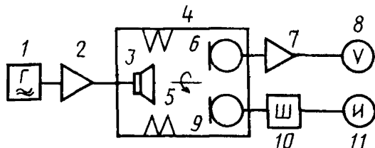
1—генератор; 2—усилитель мощности; 3—громкоговоритель; 4—заглушенная камера; 5—координатное устройство; 6—образцовый микрофон; 7—микрофонный усилитель; 8—вольтметр; 9—микрофон шумомера; 10—электрическая часть шумомера; 11—измерительный прибор шумомера
