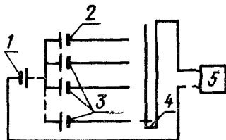
1—вспомогательный Н.Э., 2—об- разцовый Н.Э., 3—поверяемые Н.Э., 4—коммутатор Н.Э., 5—прибор для определения э.д.с.
