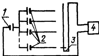
1—образцовый Н. Э.; 2—поверяемые Н. Э.; 3—коммутатор Н. Э.; 4—прибор для определения э.д.с. (потенциометр, цифровой вольтметр)
