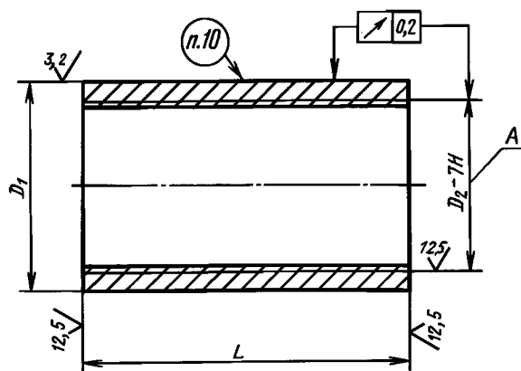
Втулка типа I
