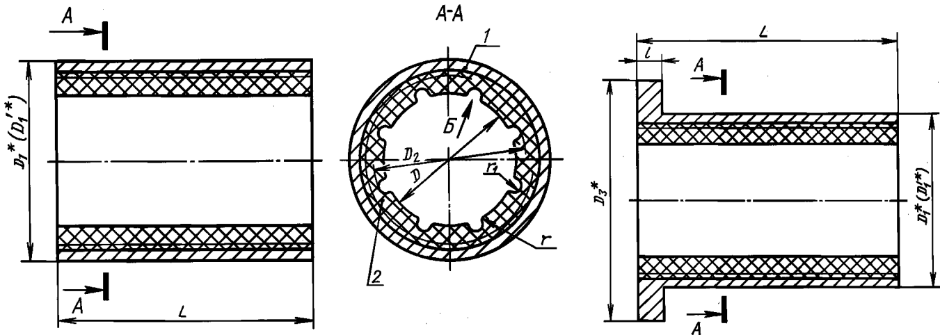
Подшипник типа I
