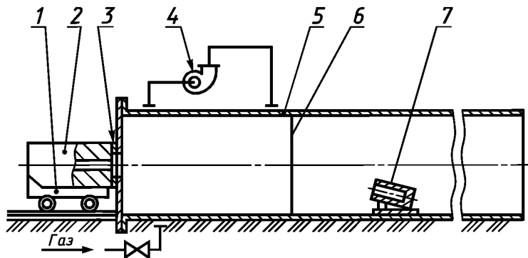
1 — тележка; 2 — канальная mortира; 3 — люк штрека; 4 — вентилятор для перемешивания метановоздушной смеси; 5 — труба штрека; 6 — диафрагма; 7 — mortира для распыления угольной пыли
