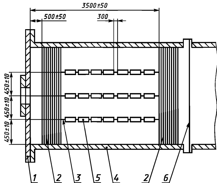
1 — дно трубы штрека; 2 — деревянная рудничная стойка; 3 — капроновая леска или провод; 4 — стенка трубы штрека; 5 — испытуемый заряд ВВ; 6 — диафрагма или штормный затвор
