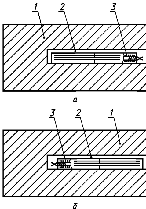
a — прямое инициирование; б — обратное инициирование 1 — канальная мортира; 2 — несквозной канал; 3 — заряд ВВ с электродетонатором
