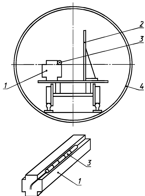
1 — уголковая мортира; 2 — отражательная стенка; 3 — испытуемый заряд ВВ; 4 — штрек
