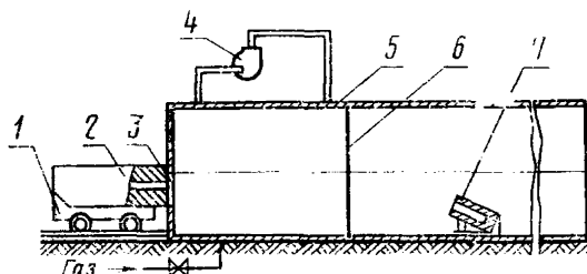
1—тележка; 2—каналная mortира; 3—люк штрека; 4—вентилятор; 5—труба штрека; 6—диафрагма; 7— распылительная mortира
