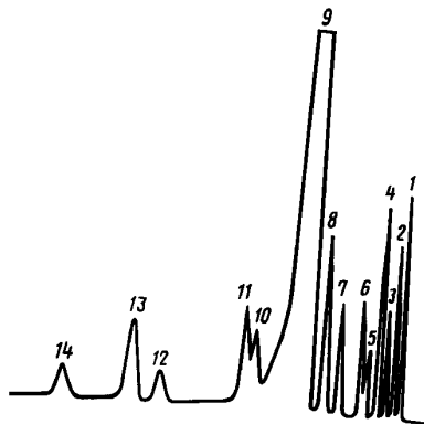
Типовая хроматограмма образца хлорбензола
